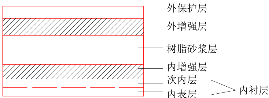
图 1 管壁结构
